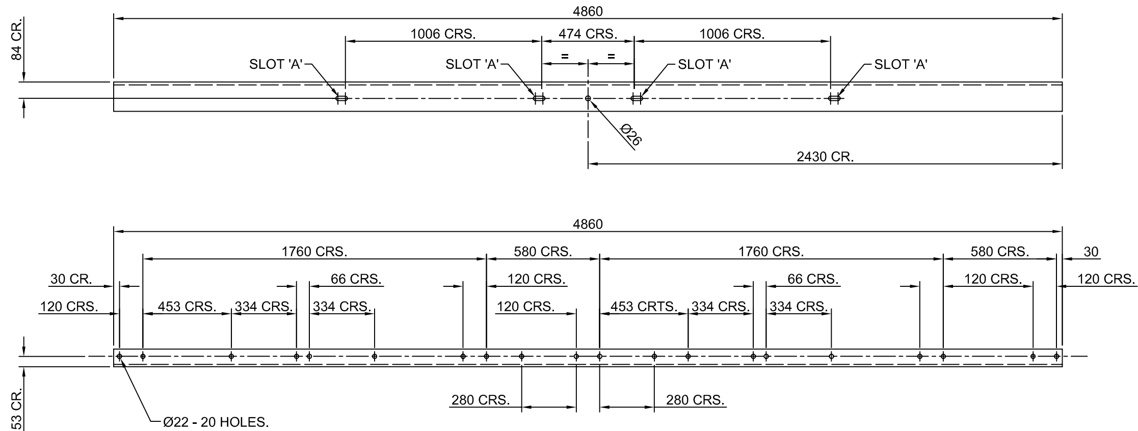
ITEM 2. 4860 LONG x 150 x 90 x 12 UNEQUAL ANGLE.
